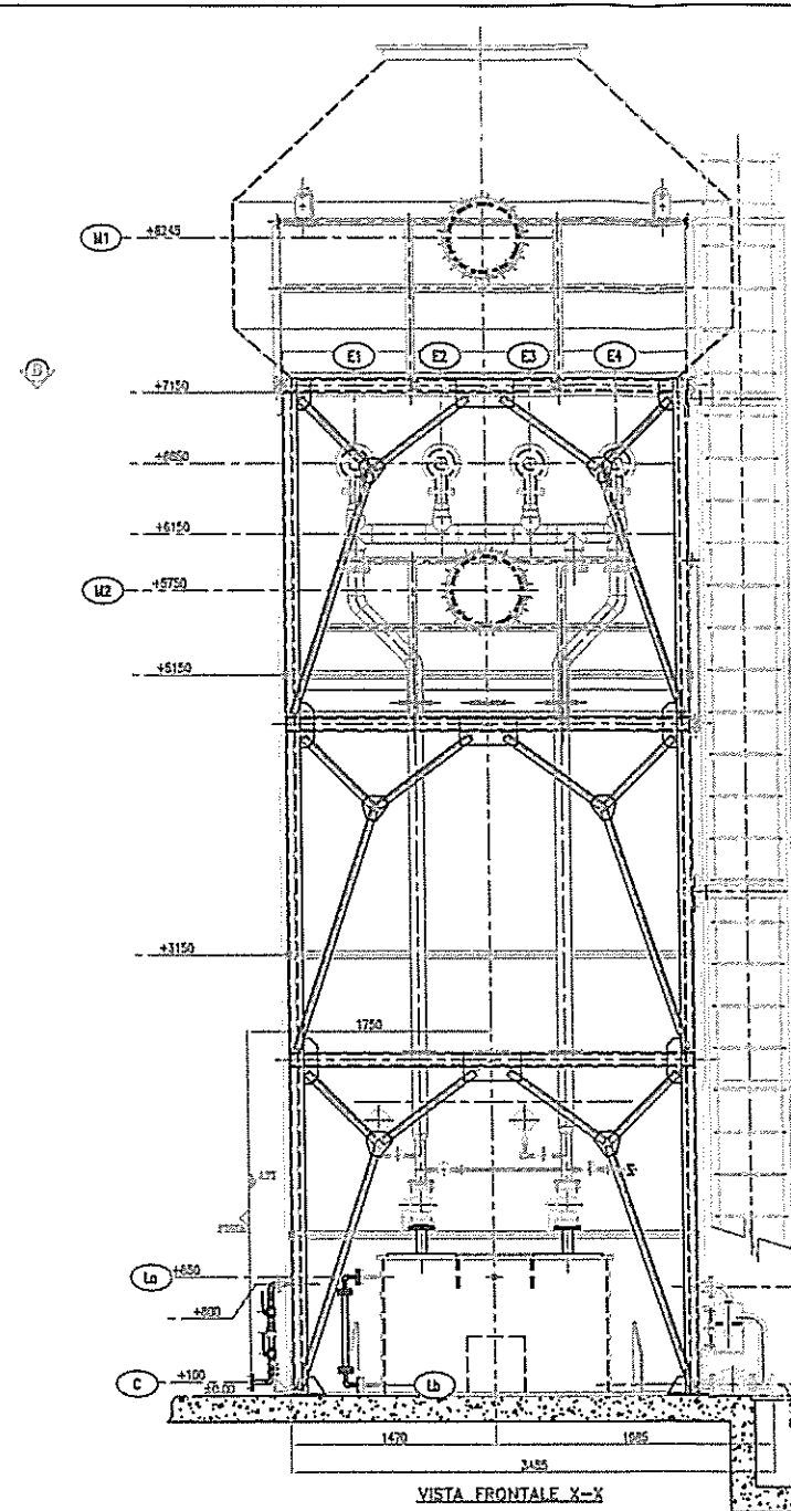
VISTA FRONTALE X-X
