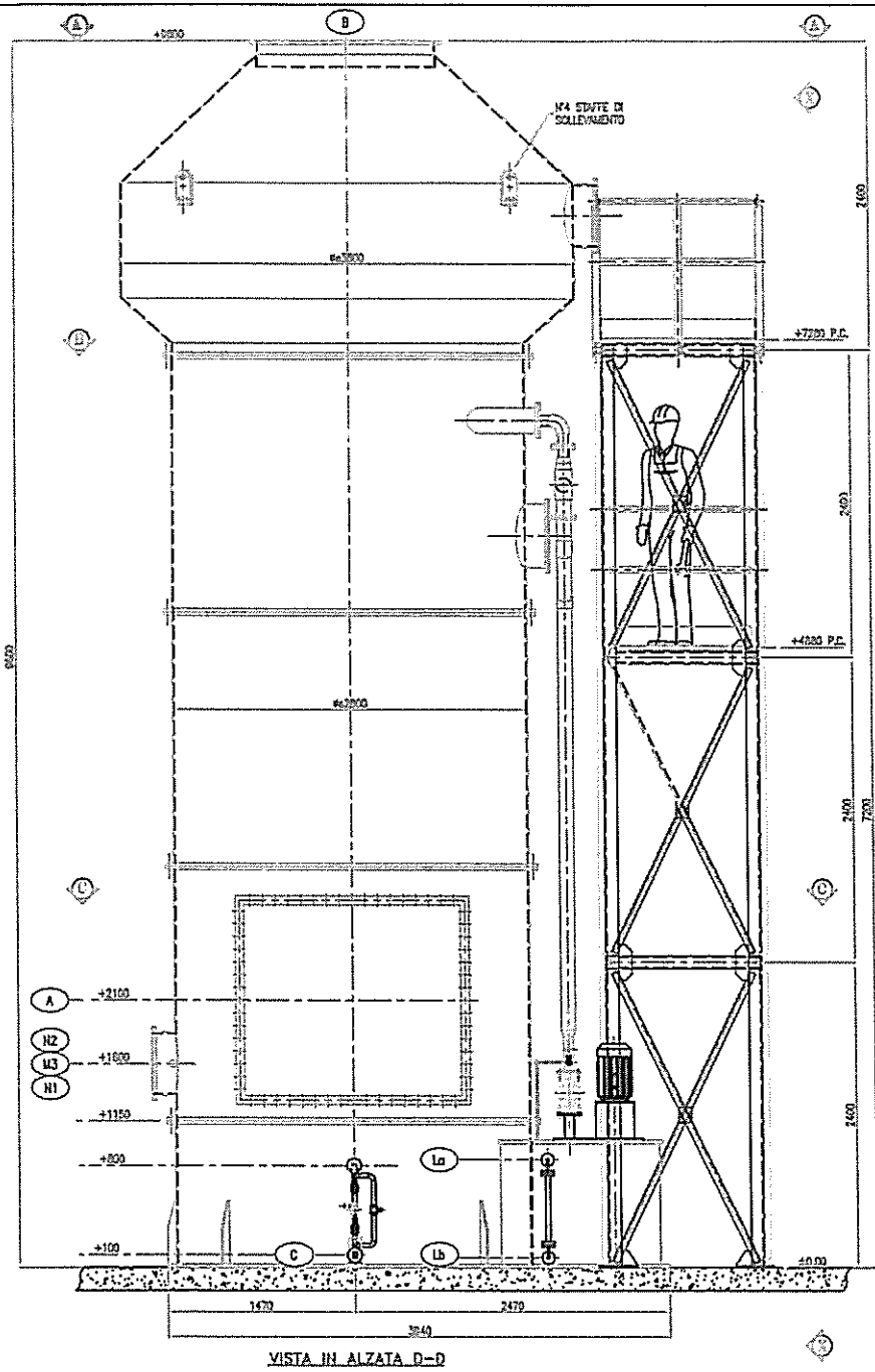
VISTA IN ALZATA D-D
